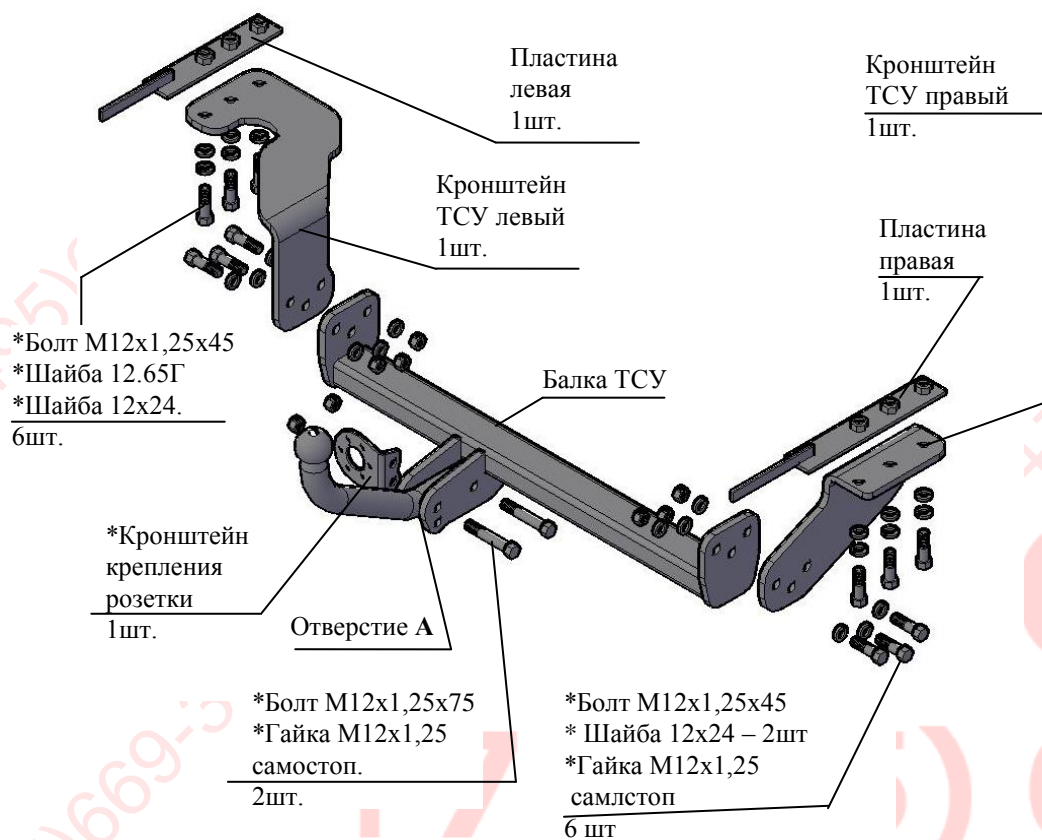
Рис.1 Тягово-сцепное устройство 7711
